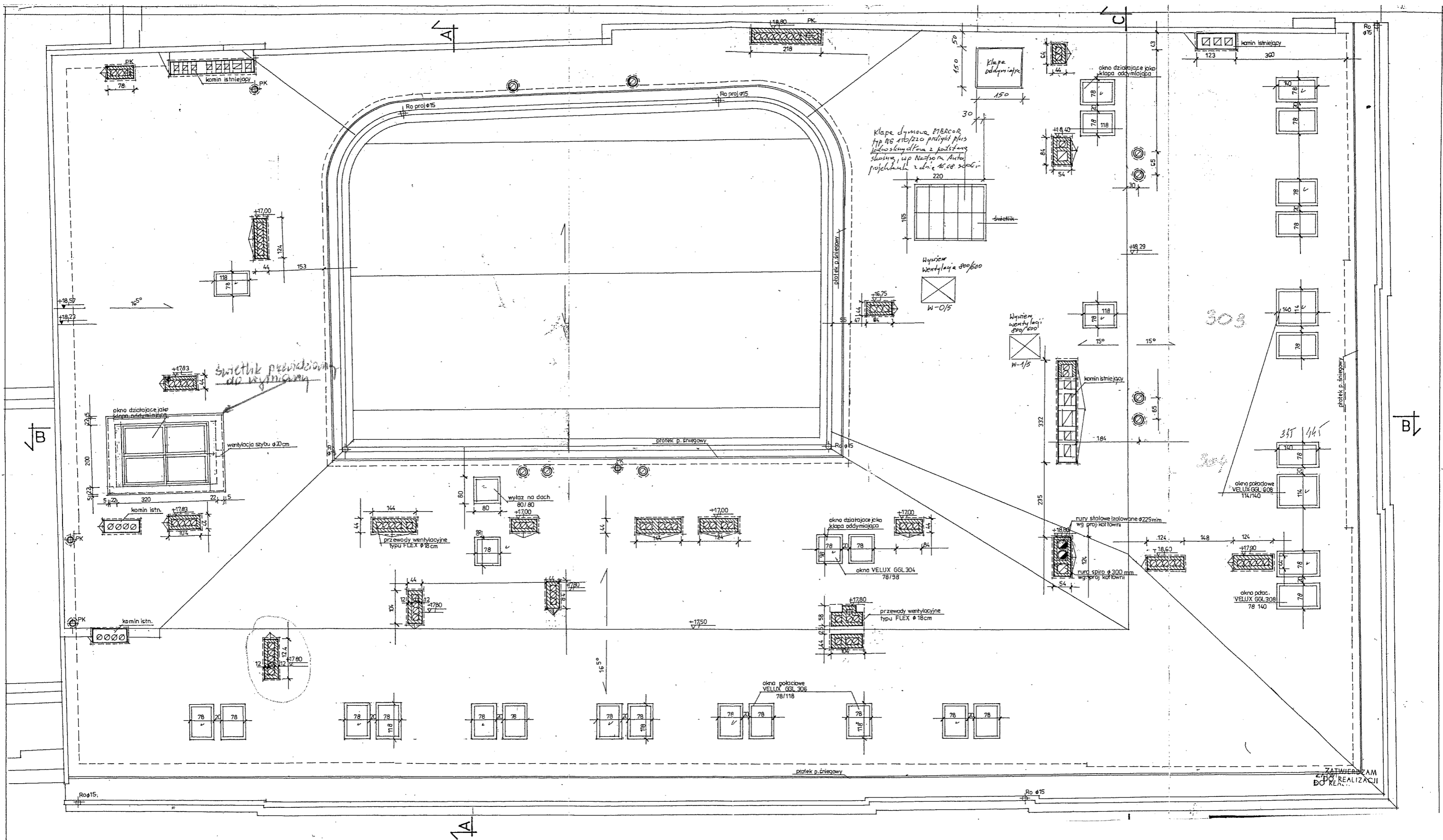
Rzut dachu budynku przy ul. Dąbnej 7 w Krakowie.
